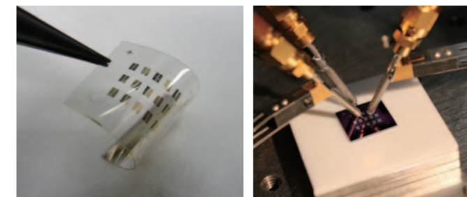
プラスチックフィルム上のトランジスタ(左)と測定の様子(右)
