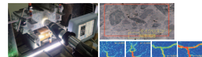
マイクロスコップを用いたコンクリートのひび割れ観察と画像解析結果
