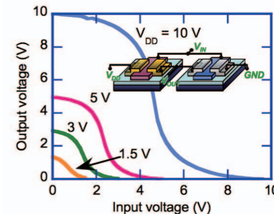
有機トランジスタと酸化物トランジスタからなる回路の特性
