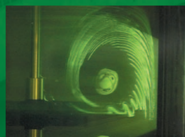
混ぜる：攪拌槽内の蛍光染料を用いた可視化
