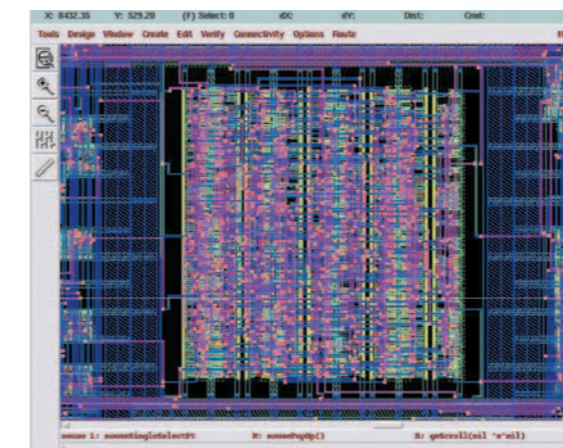
CADによるLSIレイアウト設計
