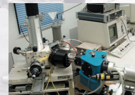
電子ビーム変調反射分光装置による新しい半導体材料の開発
